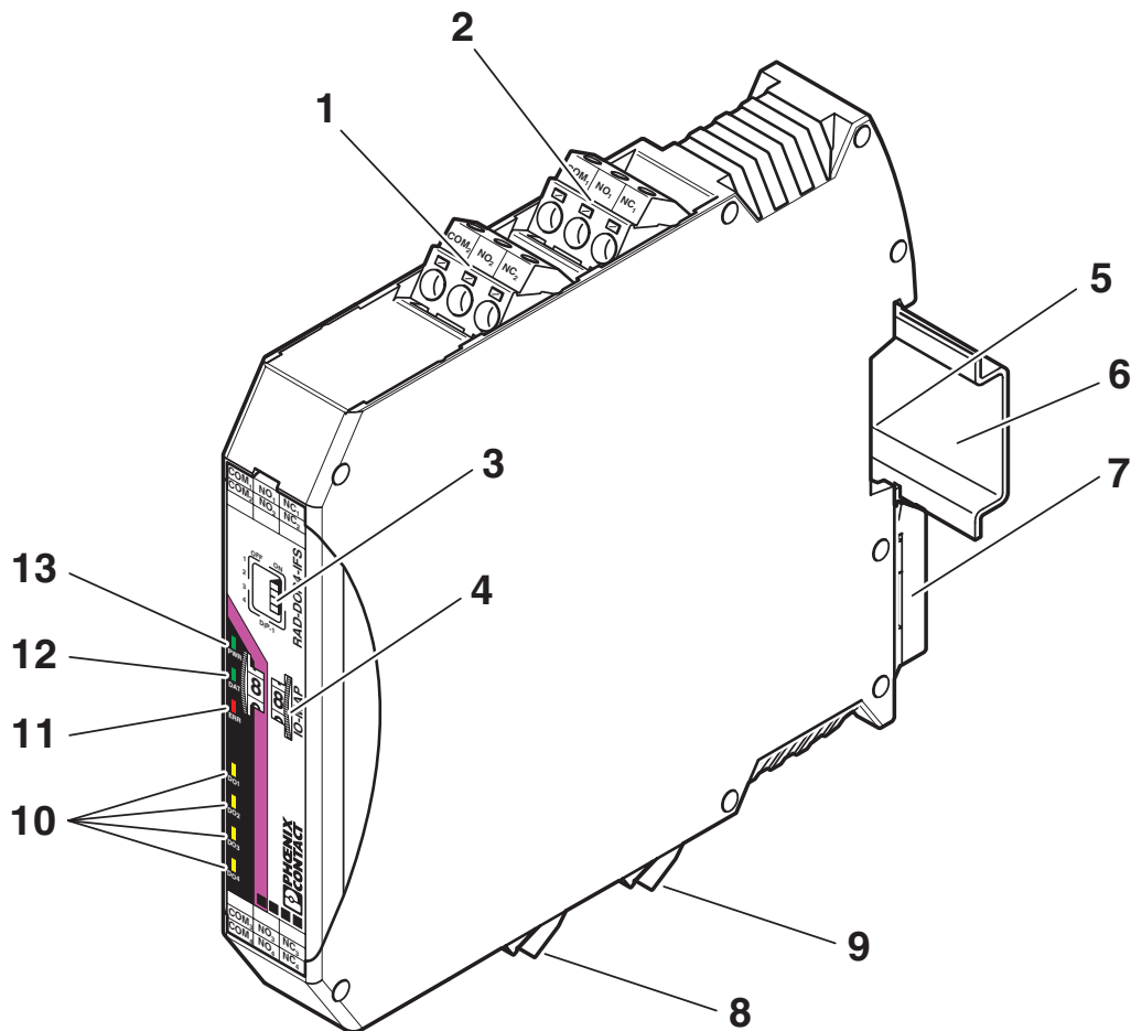
Plano esquemático
