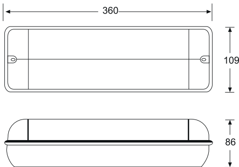
Dimensiones (mm)
