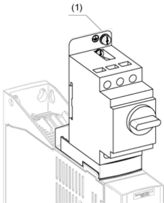
(1) Tornillo de puesta a tierra (HS tipo 2 - 5 × 12)
